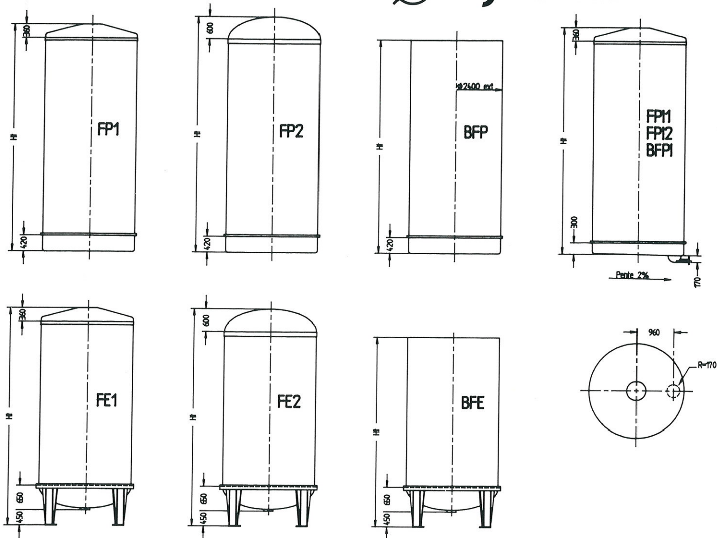
DIMENSIONS STANDARD DES CUVES EN DIAMÈTRE 2 400
